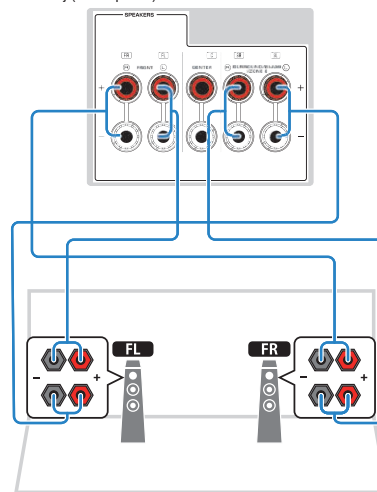
Přístroj (zadní panel)
